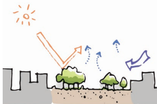
Mécanismes physiques en jeu : évapotranspiration, ombrage, absorption du rayonnement solaire ©TRIBU/ADEME
