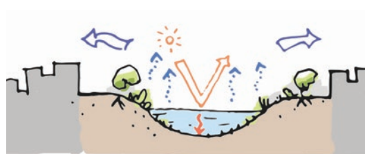
Mécanismes physiques en jeu : évaporation, vents, absorption du rayonnement solaire ©TRIBU/ADEME
